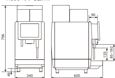
●A600マシン寸法(mm)
