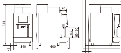
●A400マシン寸法(mm)
